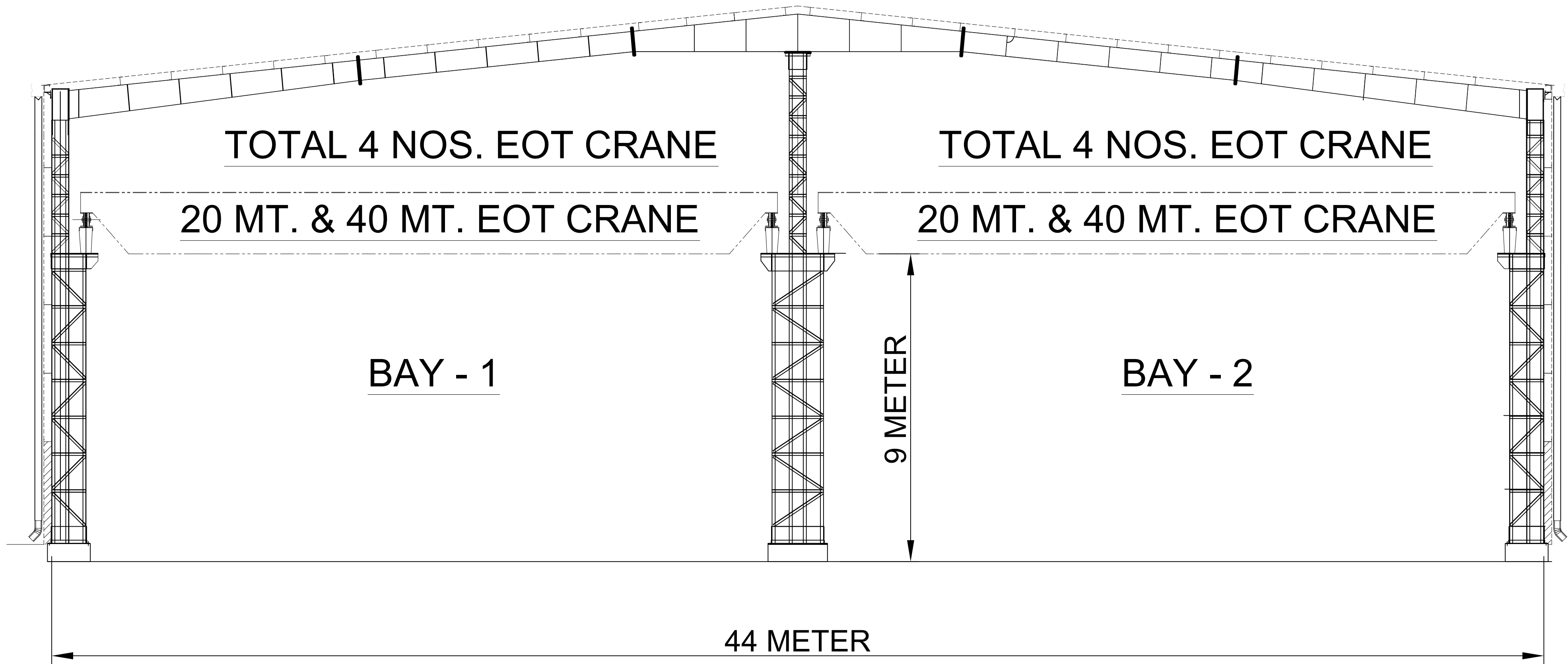
ELEVATION
